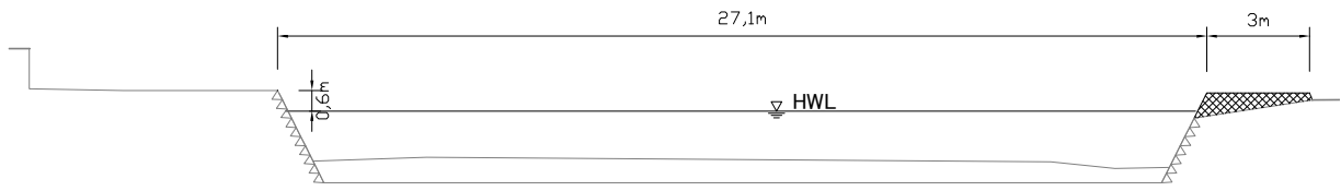
代表横断面図（鏑川合流上流約300m地点）
